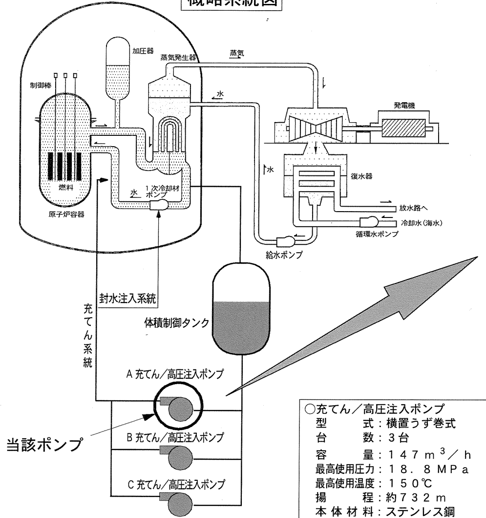
概略系統図
