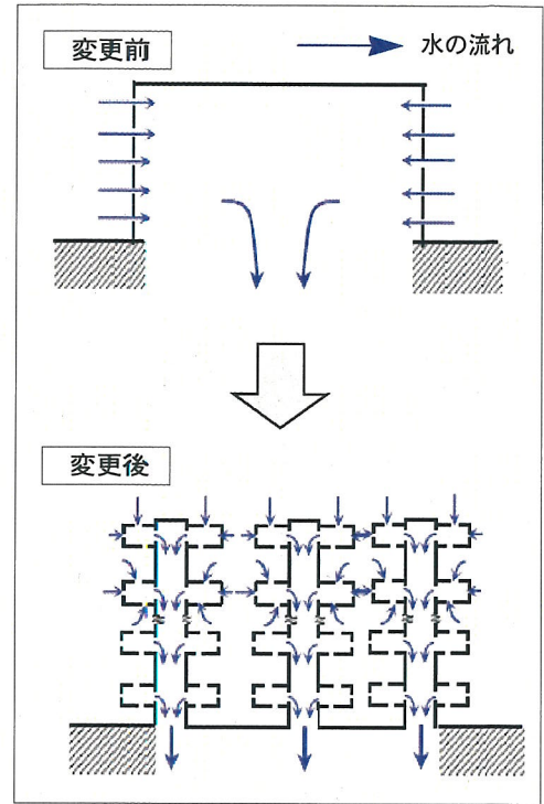
図-3 格納容器再循環サンプスクリーン取替工事
