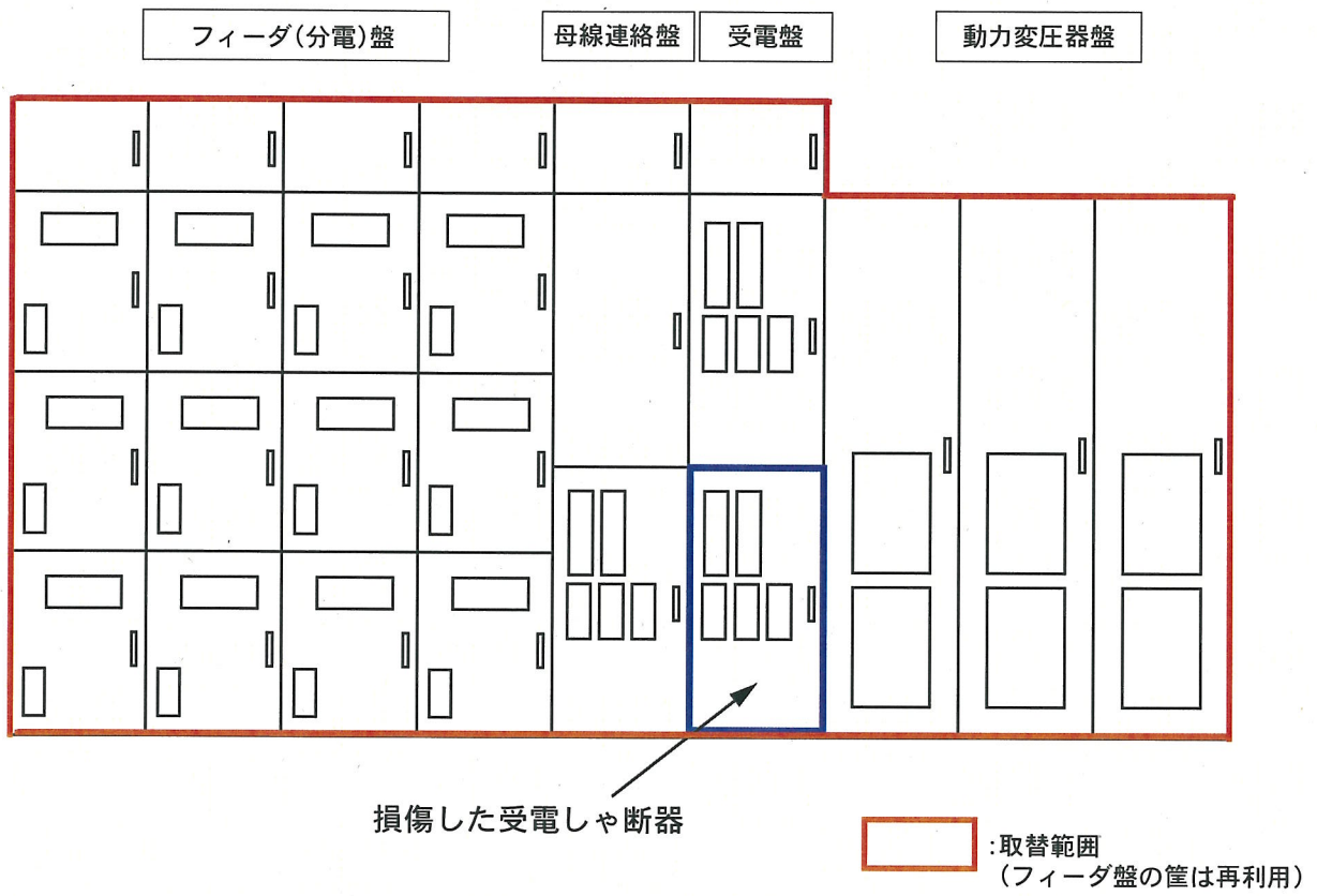
図-5 所内電源設備の取替工事
