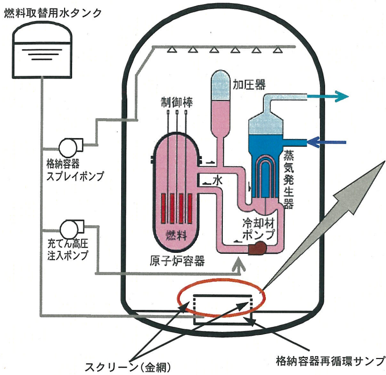
図-3 格納容器再循環サンプスクリーン取替工事
