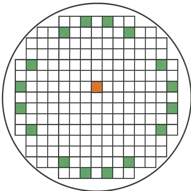
燃料集合体装荷位置図
