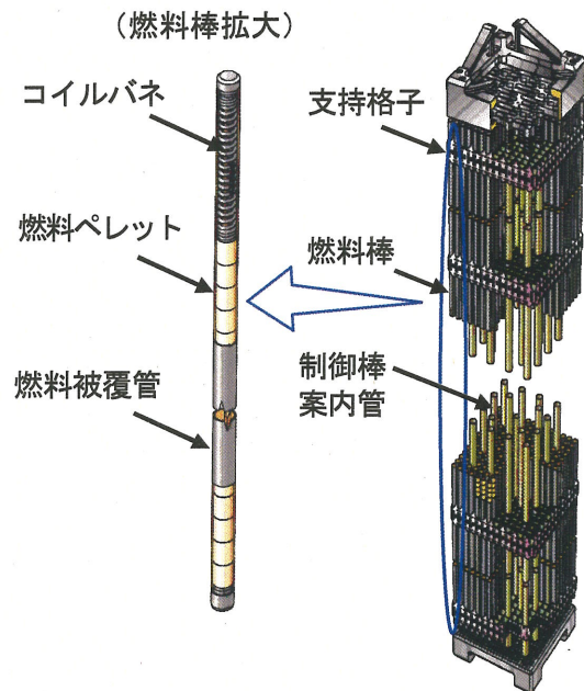
○漏えい燃料集合体の仕様概要
