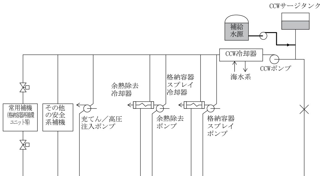
【4-3：補機冷却水系回復】
