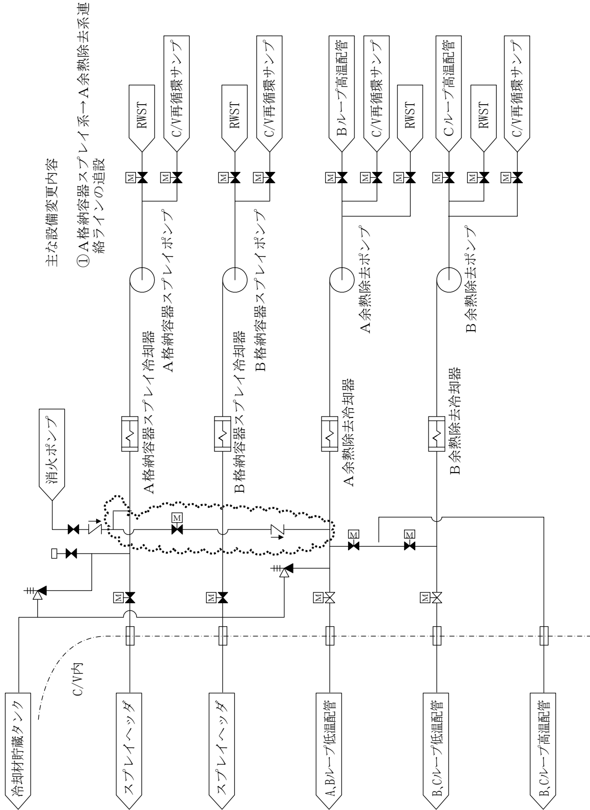
川内2号機 設備変更を実施した防護措置の概略図 (代替再循環)
