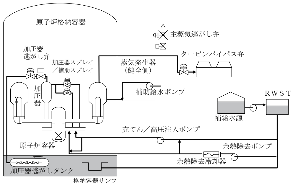
【2-15：クールダウン&リサーキュレーション】
