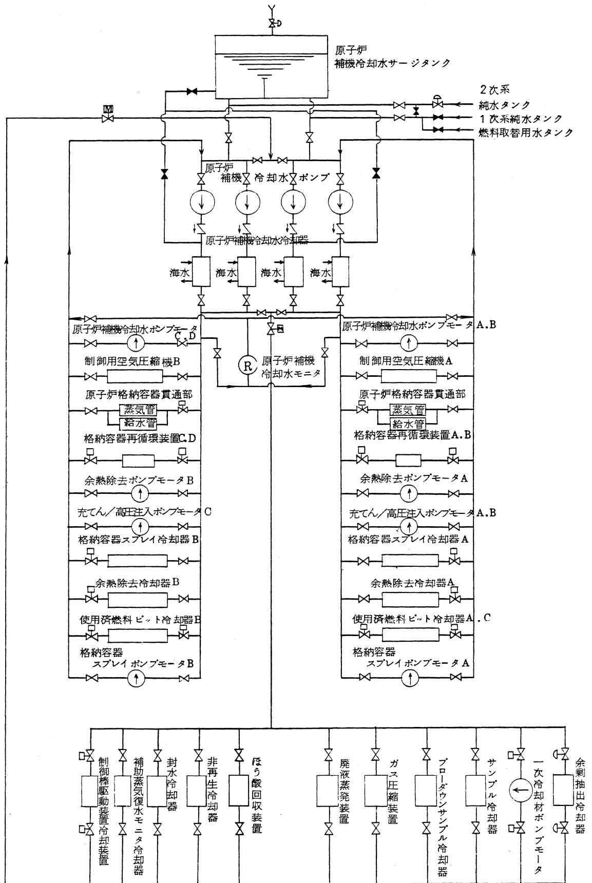
川内 2 号機の系統構成 (補機冷却水系)
