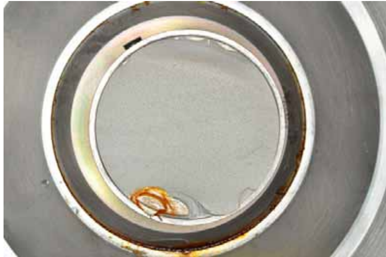
主軸の折損状況（折損部断面）
