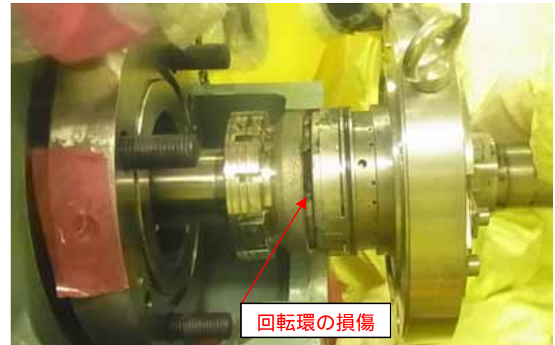
メカニカルシールの損傷状況
