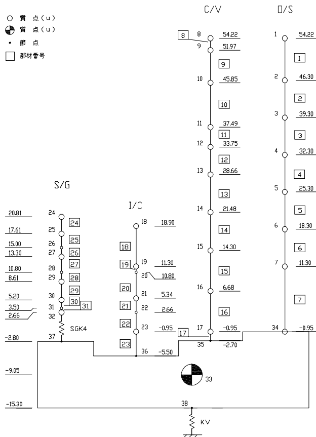
図 2-2 原子炉建屋の解析モデル (鉛直)
