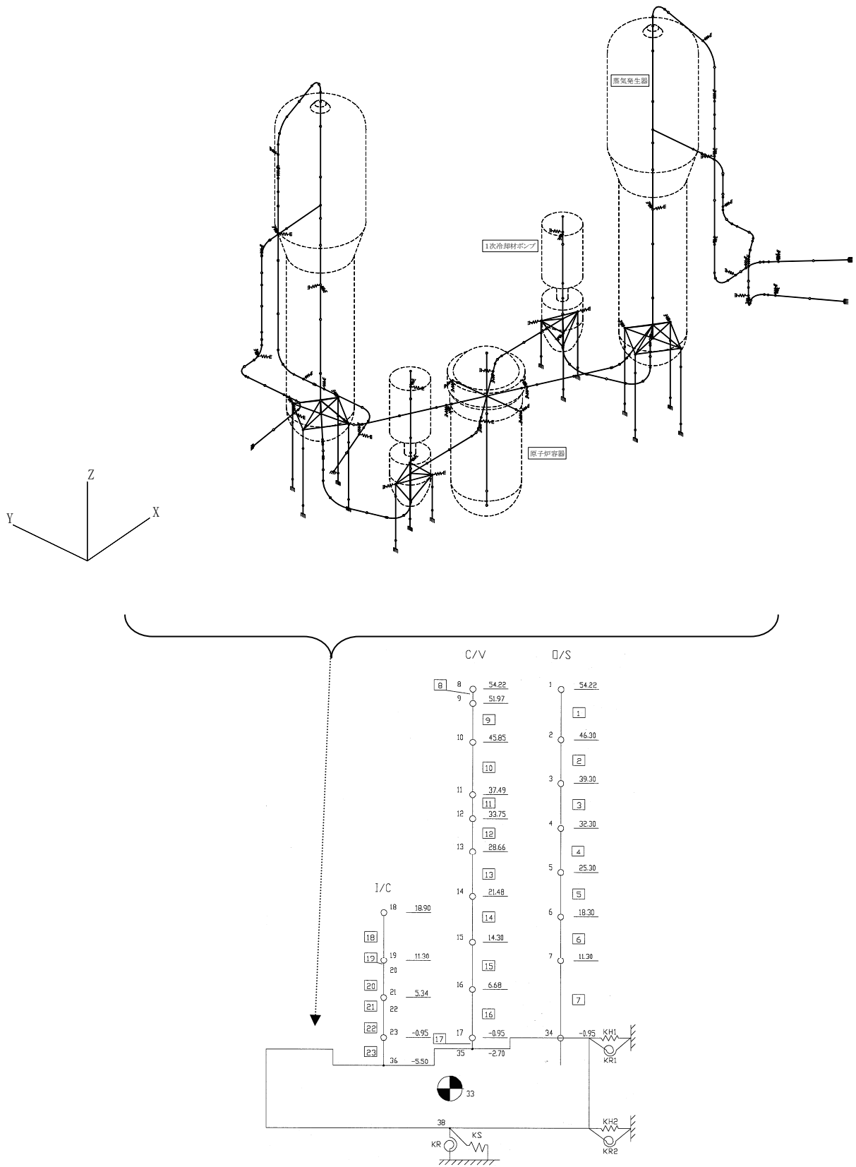
図 3-3 1次冷却設備の建屋-機器連成解析モデル (例: 水平方向)
