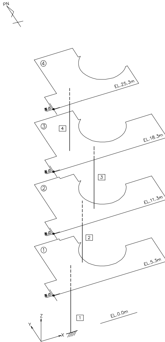
図 2-3 原子炉補助建屋の解析モデル (水平)
