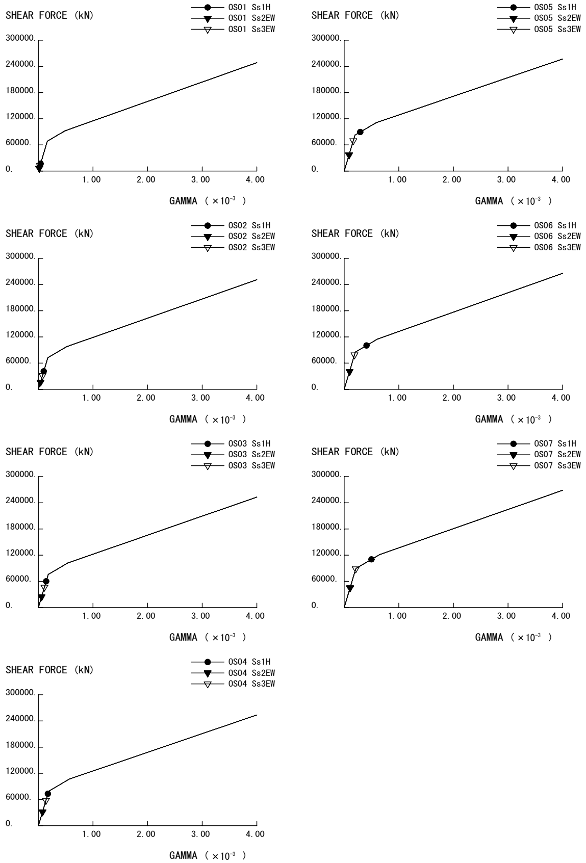
図 2 - 5 - 3 Q- \gamma 関係と最大応答値 (原子炉建屋 OS EW 方向)
