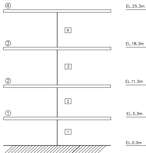
図 2-4 原子炉補助建屋の解析モデル (鉛直)
