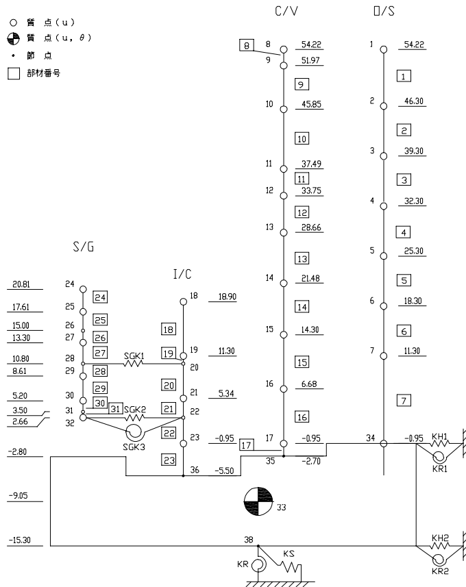
図 2-1 原子炉建屋の解析モデル (水平)
