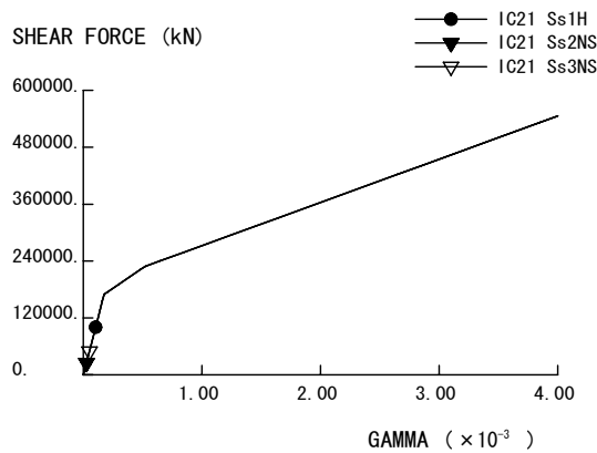
図 2-5-2 Q- \gamma 関係と最大応答値 (原子炉建屋 IC NS 方向)
