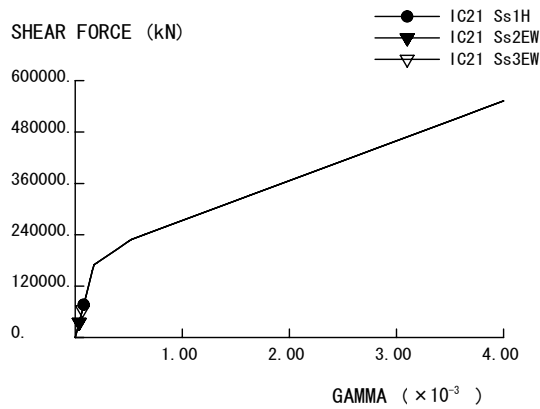
図 2-5-4 Q- \gamma 関係と最大応答値 (原子炉建屋 IC EW 方向)
