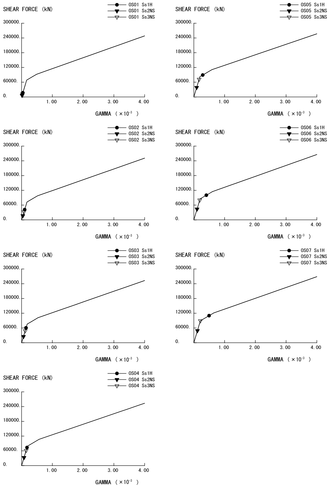
図 2-5-1 Q- \gamma 関係と最大応答値 (原子炉建屋 OS NS 方向)
