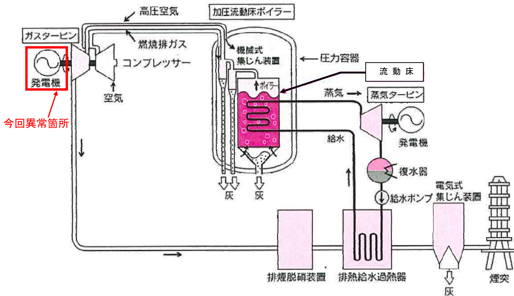
[荻田発電所新第1号機 概略図]
